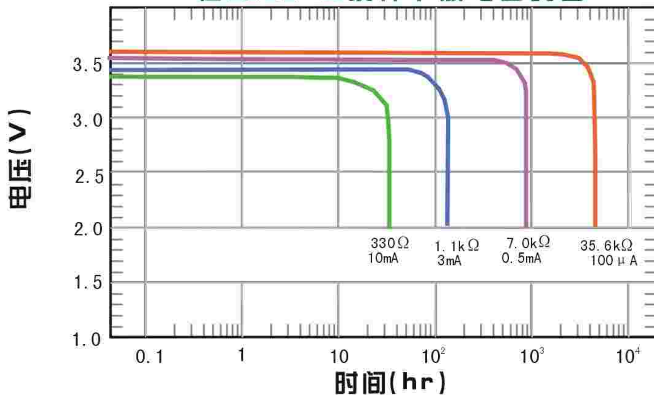
在 23±2 °C 条件下放电曲线图
