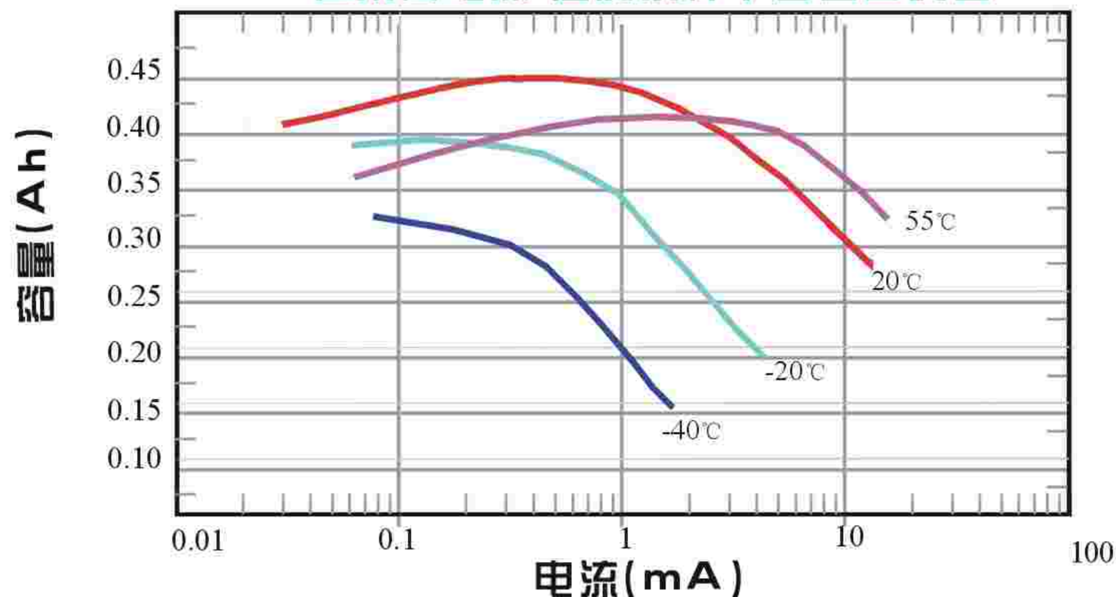
在不同电流,温度条件下容量曲线图
