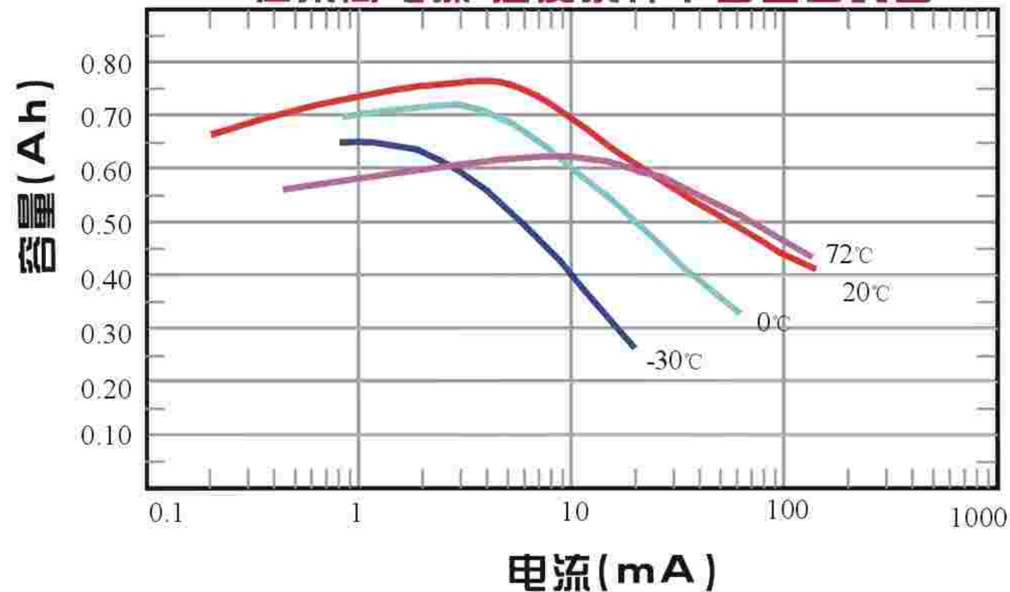
在不同电流,温度条件下容量曲线图
