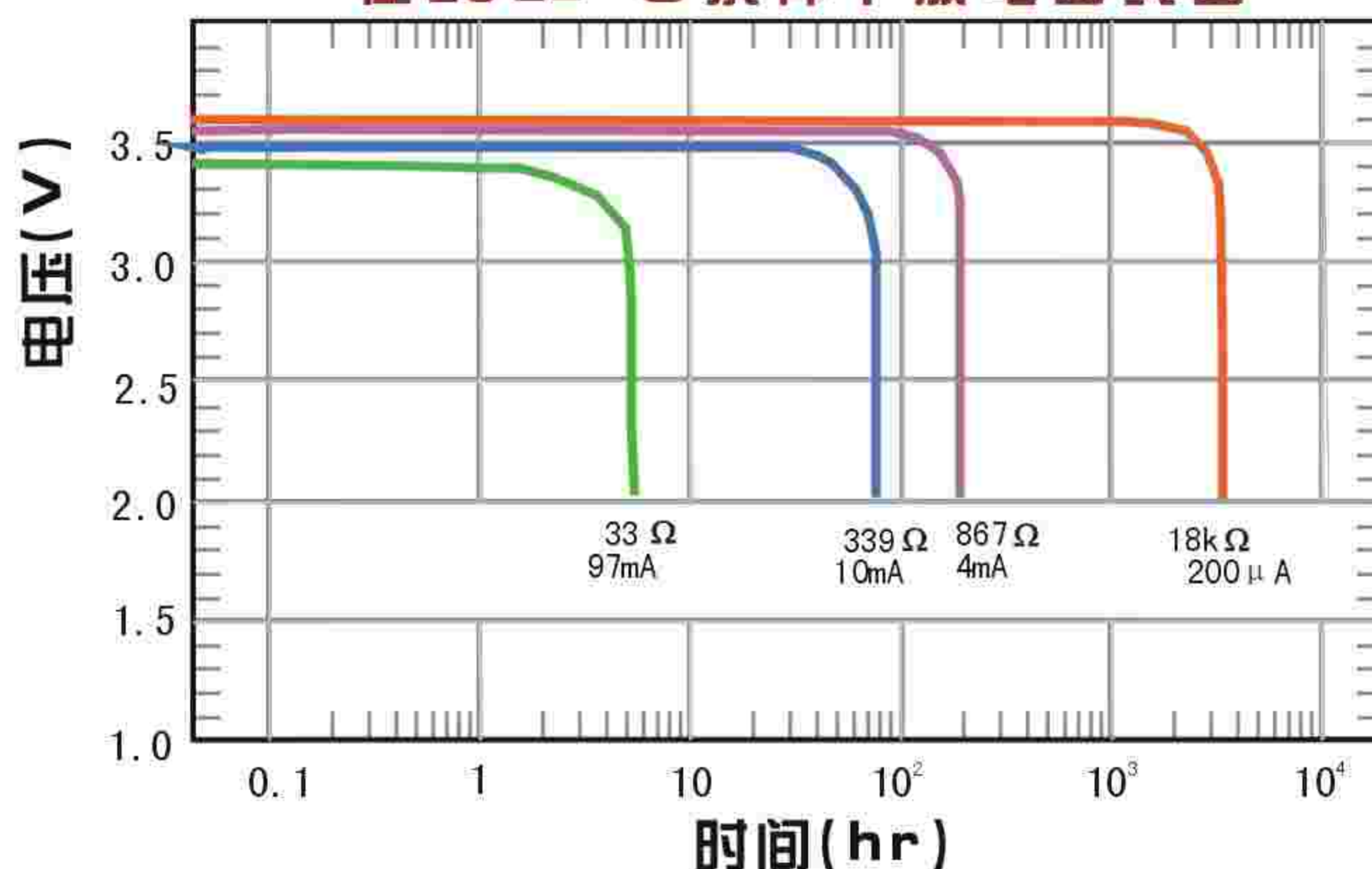
在 23 \pm 2^{\circ}\text{C} 条件下放电曲线图
