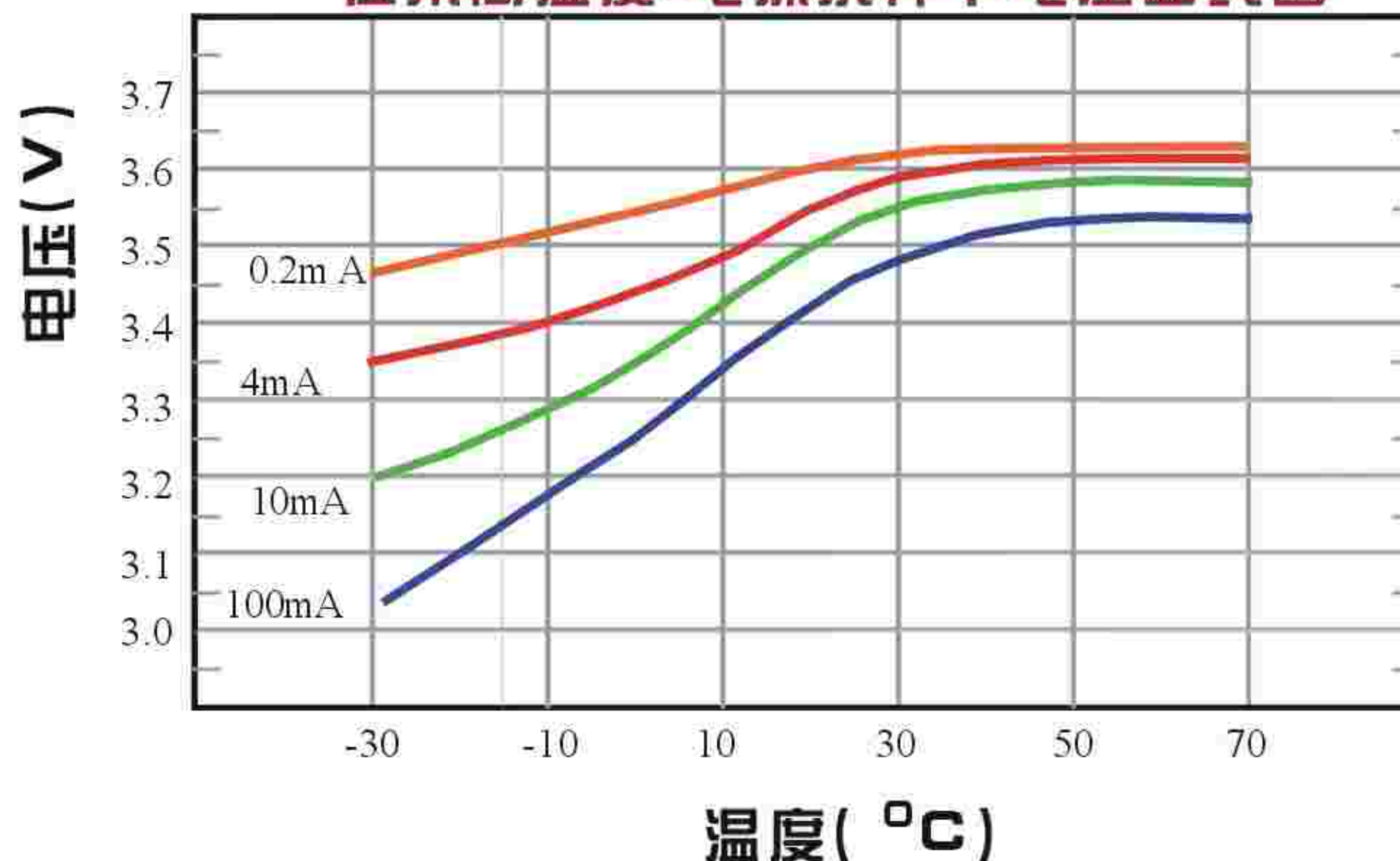
在不同温度,电流条件下电压曲线图
