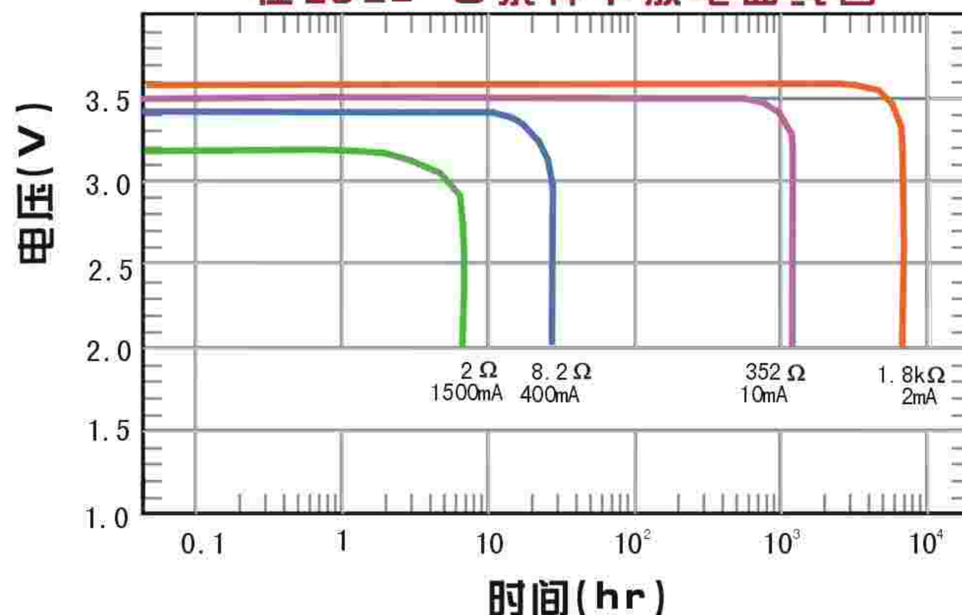
在不同电流,温度条件下容量曲线图
