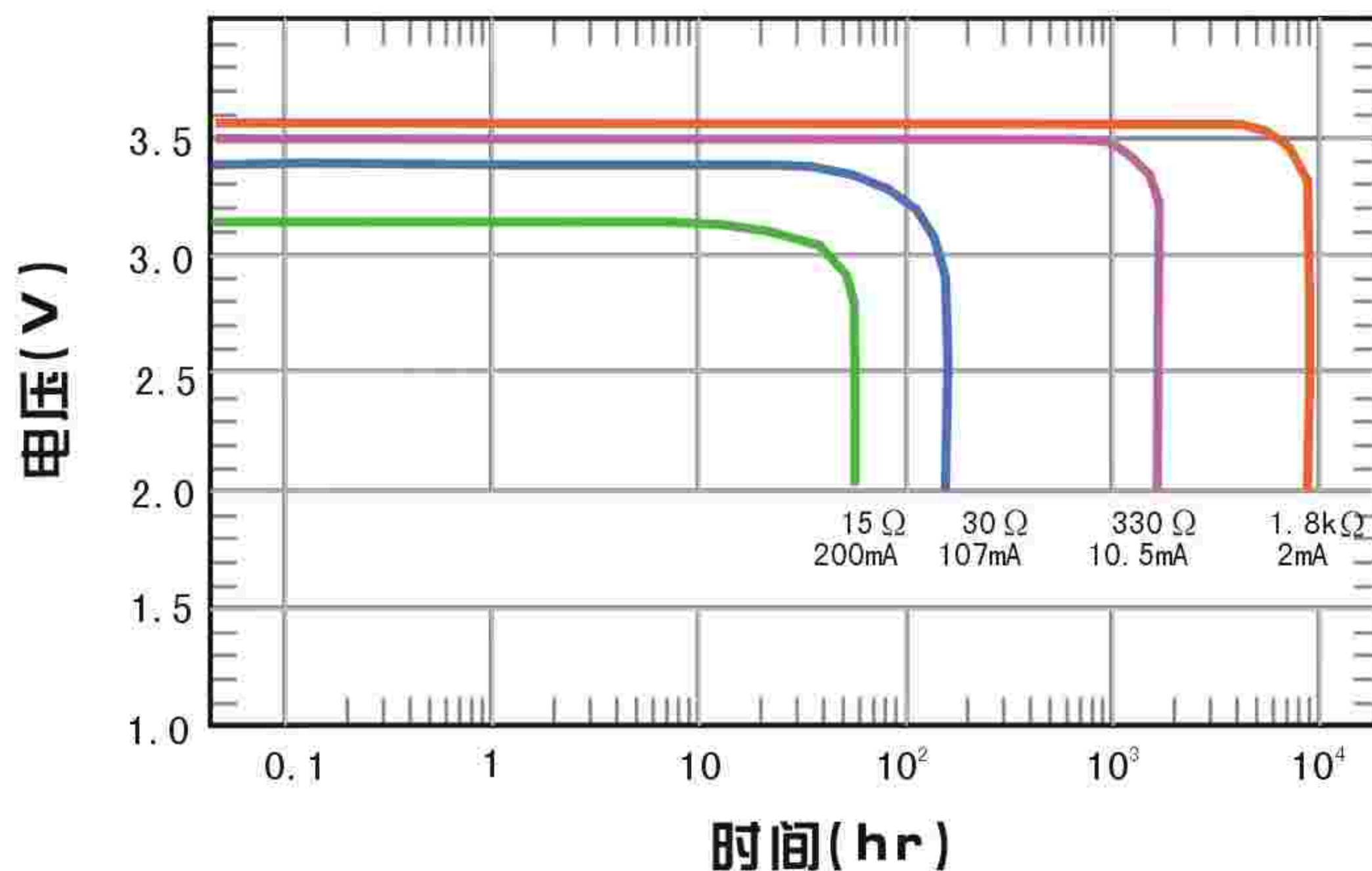
在 23 \pm 2^{\circ}\text{C} 条件下放电曲线图
