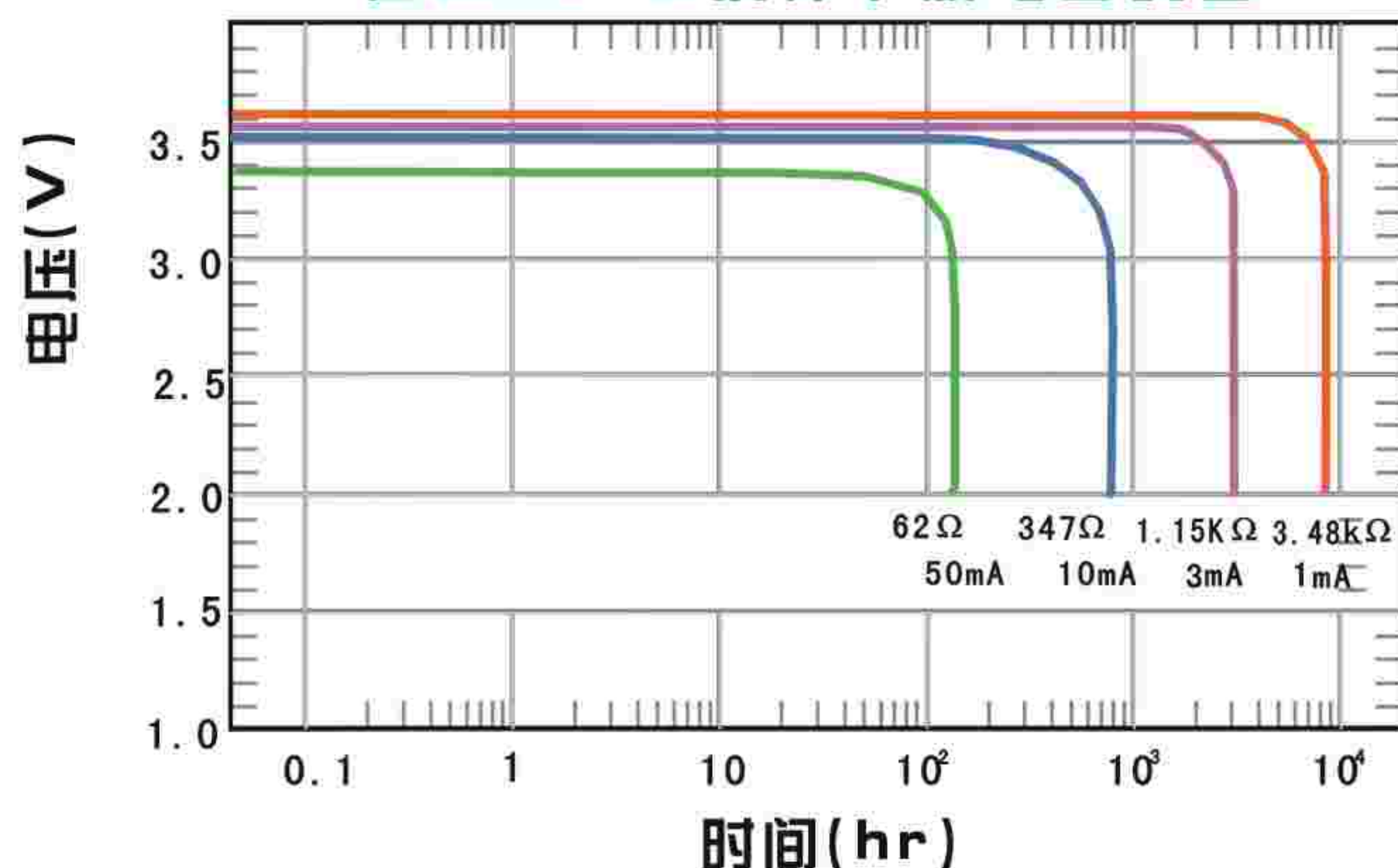
在 23±2 °C 条件下放电曲线图
