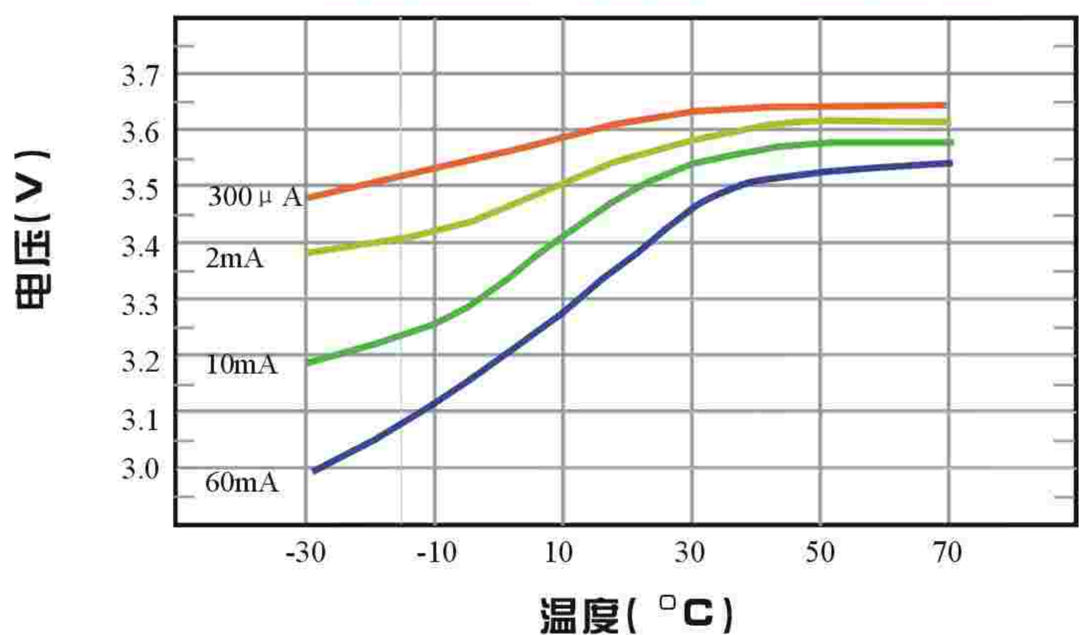
在不同温度,电流条件下电压曲线图
