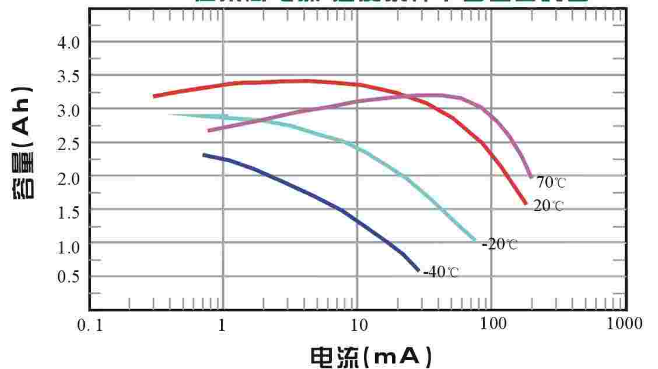
在不同电流,温度条件下容量曲线图
