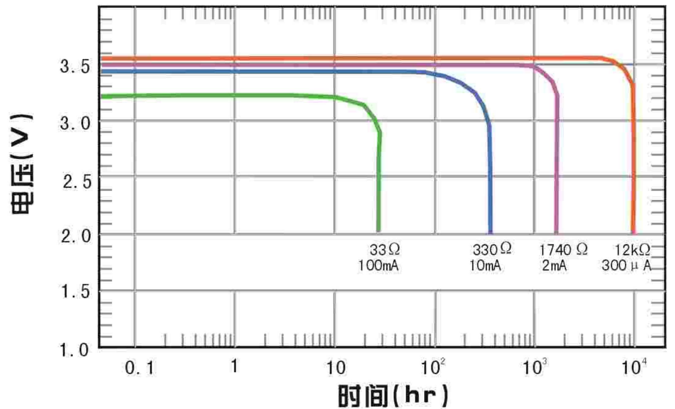
在 23±2 °C 条件下放电曲线图
