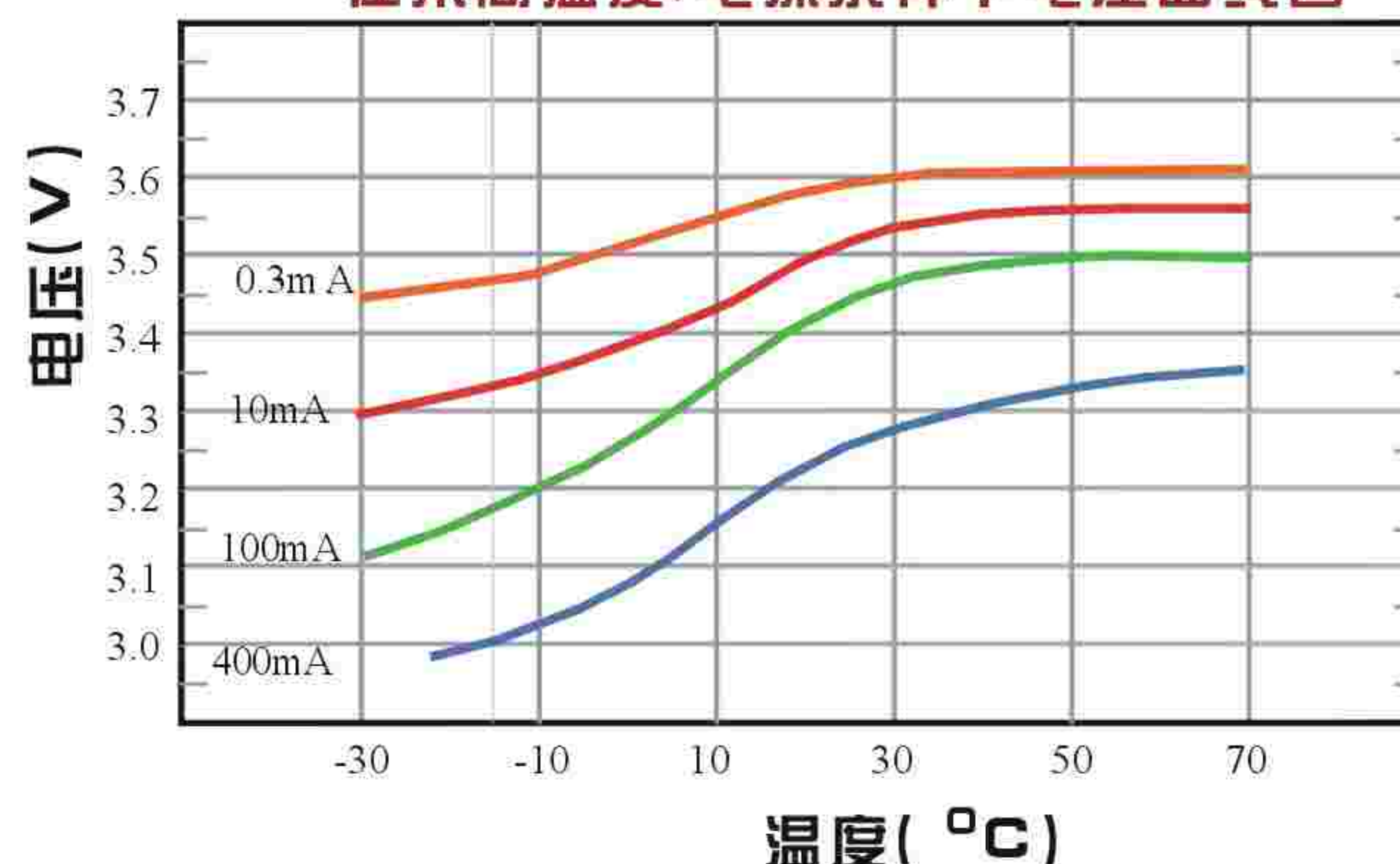
在不同温度,电流条件下电压曲线图
