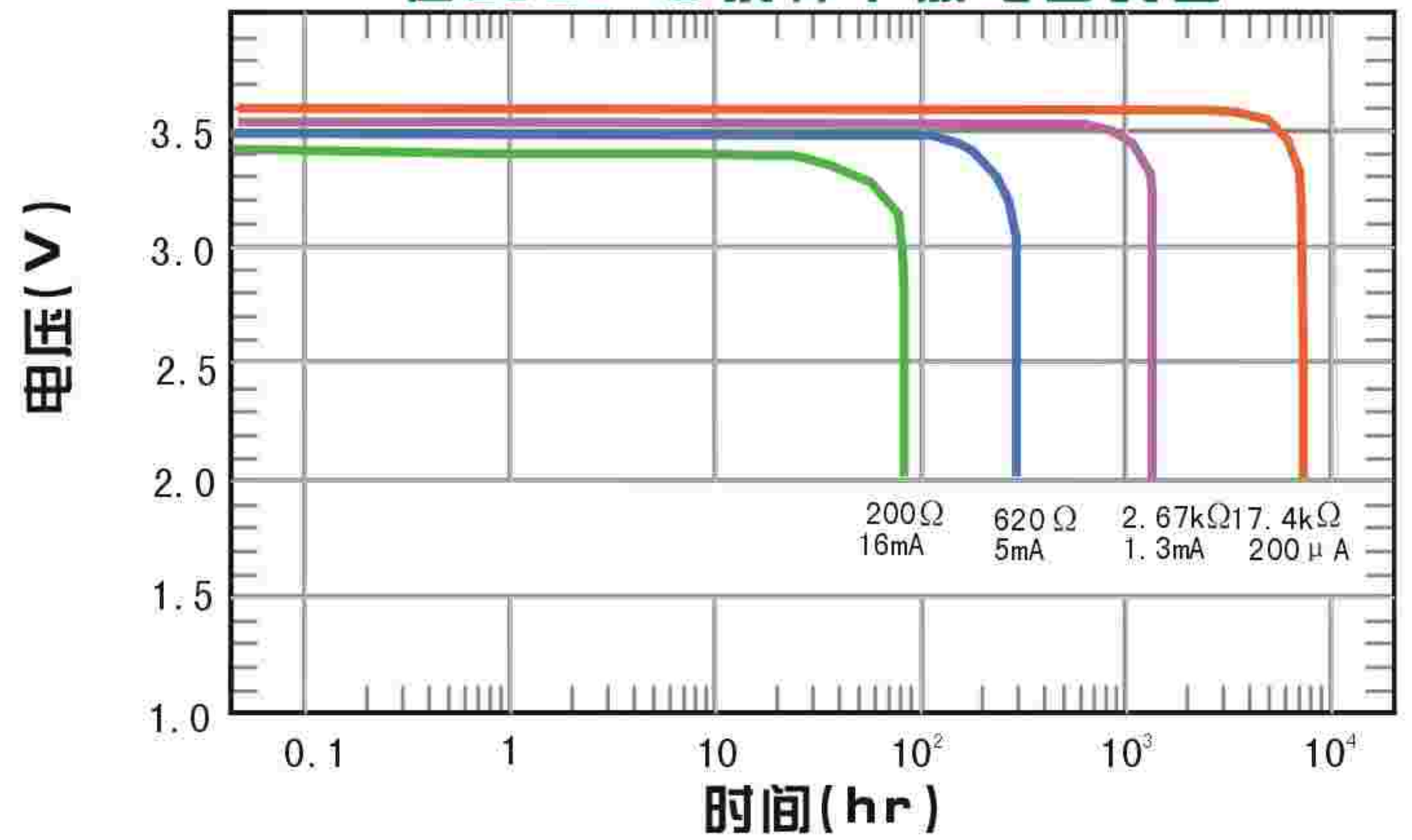
在不同电流,温度条件下容量曲线图
